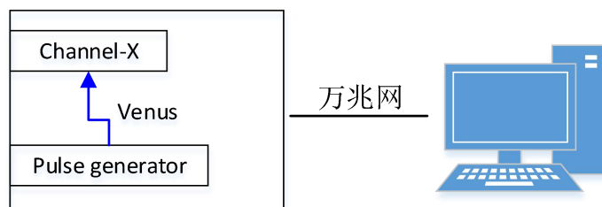
图 104 双通道时间差测量示意图（内部触发）
