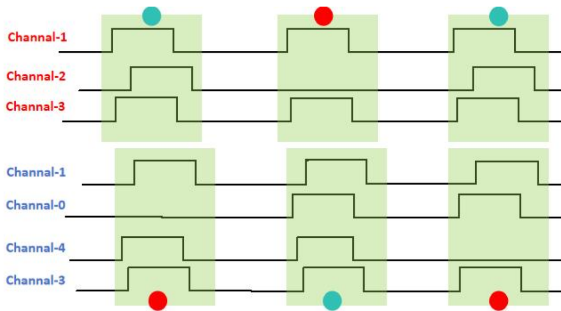
图 76 多重符合示意图（以 2 个策略组，3/4 重符合为例）
