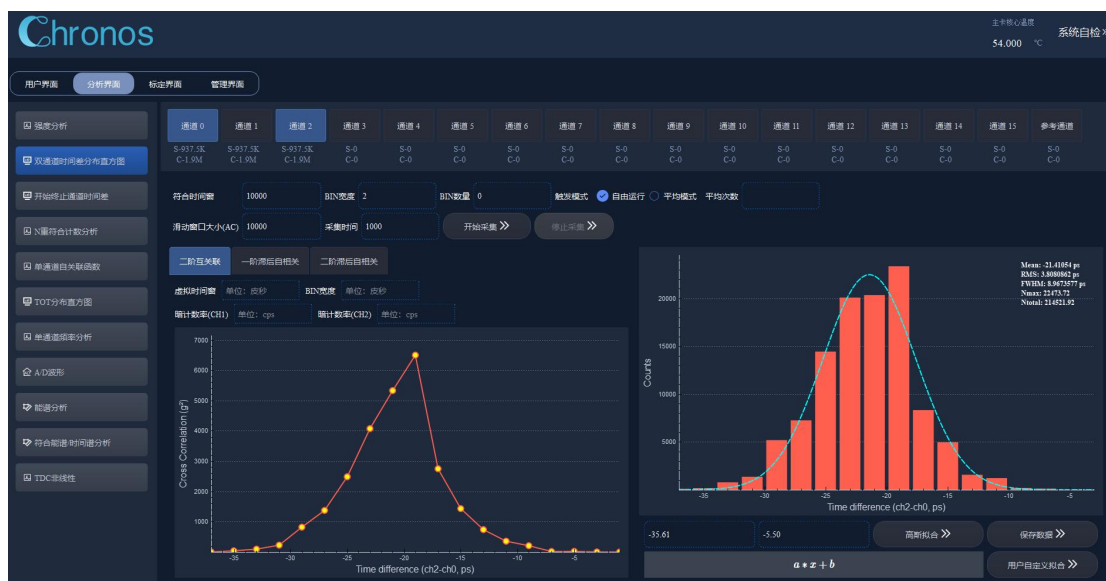
图 105 高分辨率通道双通道时间差分布直方图典型测试结果（内部触发，上升沿，CH0/2）
