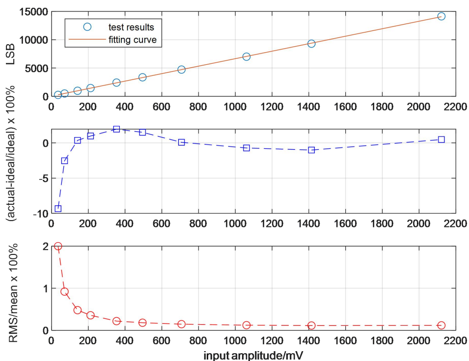
图 137 能量测量线性和分辨率测试典型结果（通道 1）
