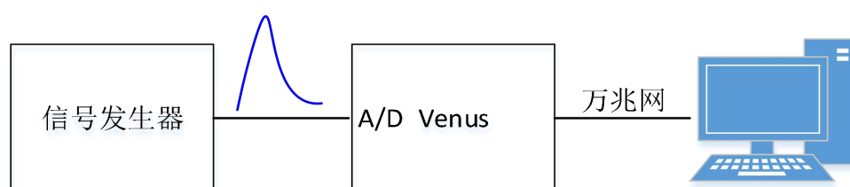
图 121 模拟-数字转换实时波形测量
