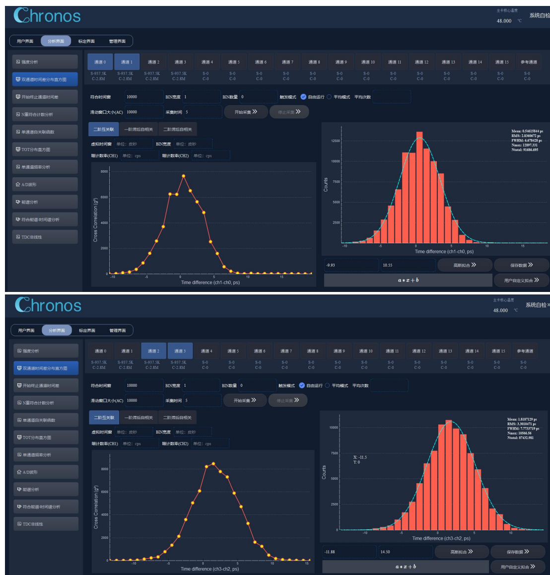
图 108 Venus Lite4-2ps 特殊版本双通道时间晃动测试（内部触发，上图：通道 0 和通道 1，下图：通道 2 和通道 3）
