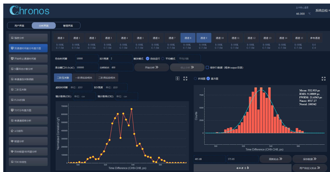
图 111 双通道时间差外部输入信号测量结果（普通通道，通道 8 和 9，上升沿，典型结果）
