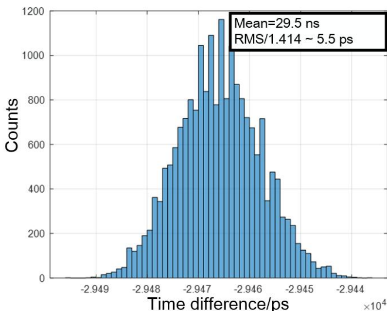
图 143 双板通道间的时间差分布直方图典型测试结果
