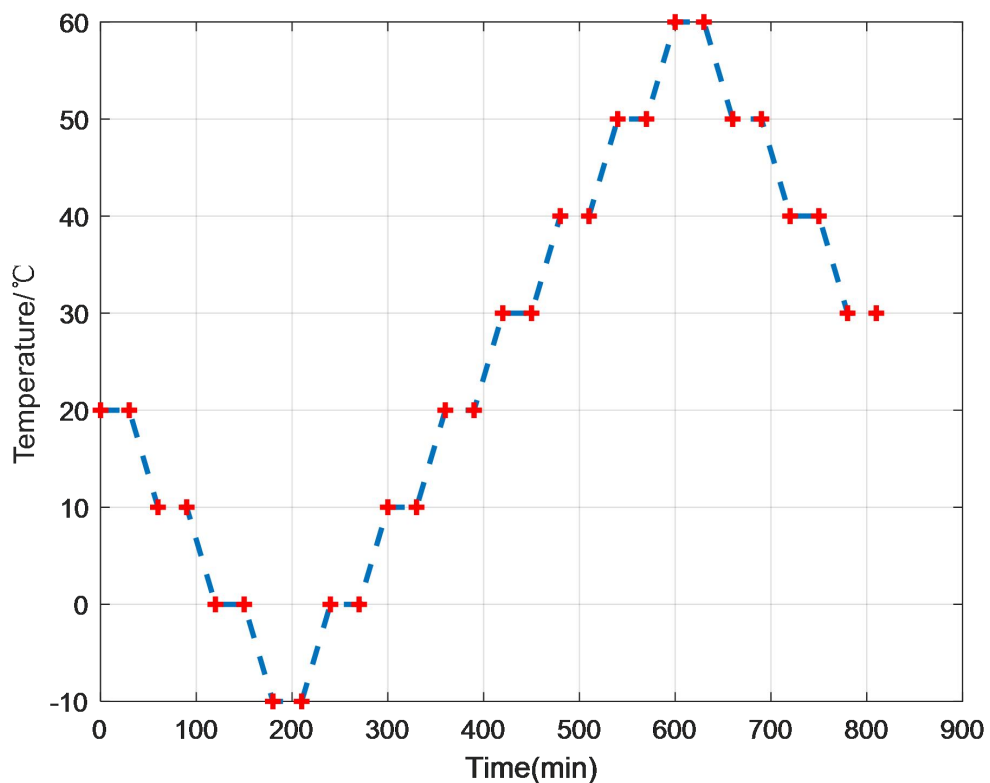
图 131 温度循环实验温度曲线设置
