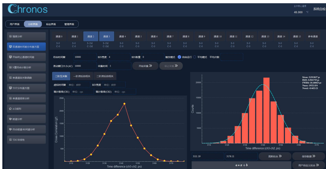
图 113 Venus Lite4-2ps 特殊版本双通道时间晃动测试（外部触发，上图：通道 0 和通道 1，下图：通道 2 和通道 3）
