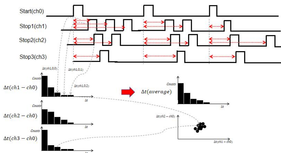
图 58 Start-stop 统计示意图（以上升沿触发为例，以 CH0 作为 start 通道，CH1/2/3 为 Stop 通道为例。实际用户可以按照实验要求自行分组）
