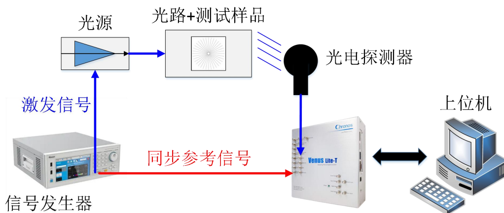
图 61 一种常见的 Start-stop 功能应用测试场景
