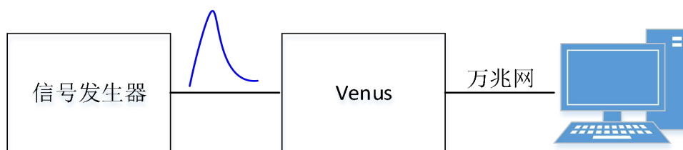
图 114 单通道周期信号重复频率测量示意图
