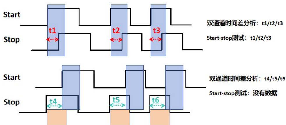
图 145 双通道时间差与 Start-stop 测试区别示意图（上升沿触发举例）。
