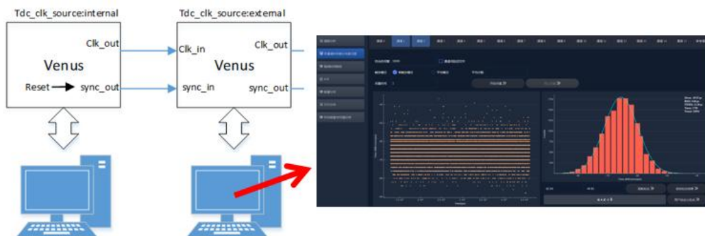
图 134 2 台 Venus 设备串联，第二台设备使用外部时钟进行时间晃动测试（内部触发）
