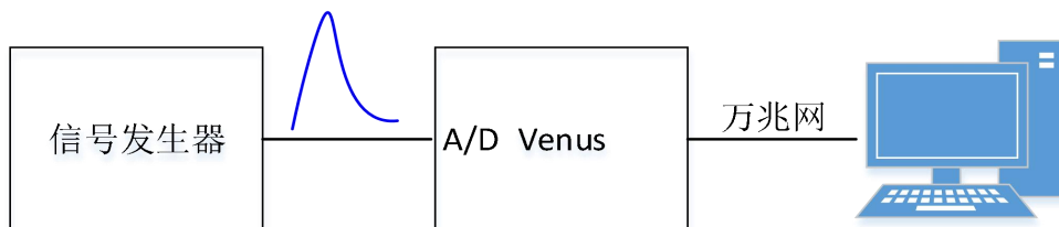
图 125 能谱测量示意图
