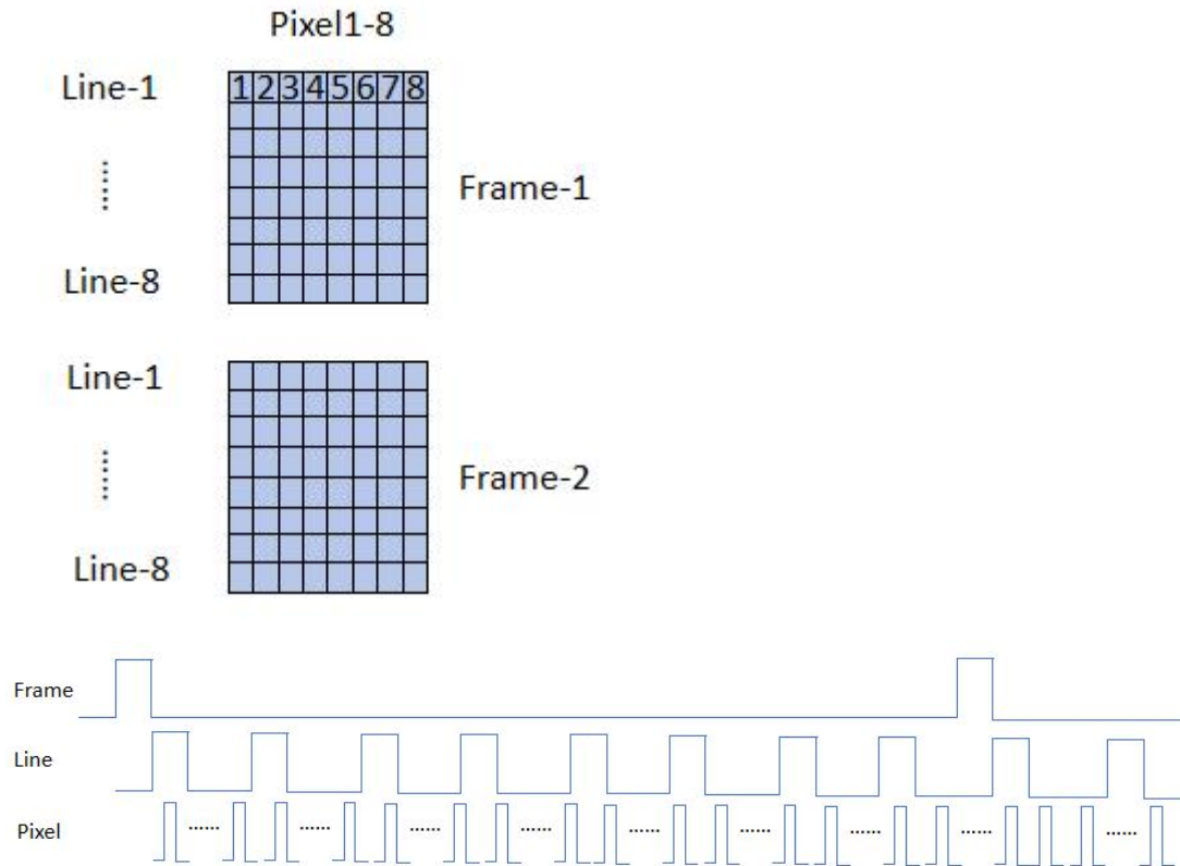
图 81 同步扫描位置信号（Frame/Line/Pixel 示意图，以 2 帧，8x8 图像为例）
