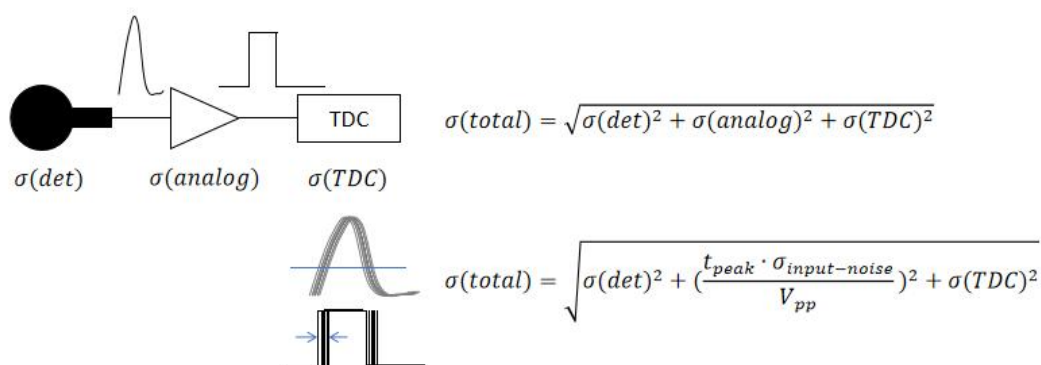
图 146 一般测量系统时间晃动分析模型
