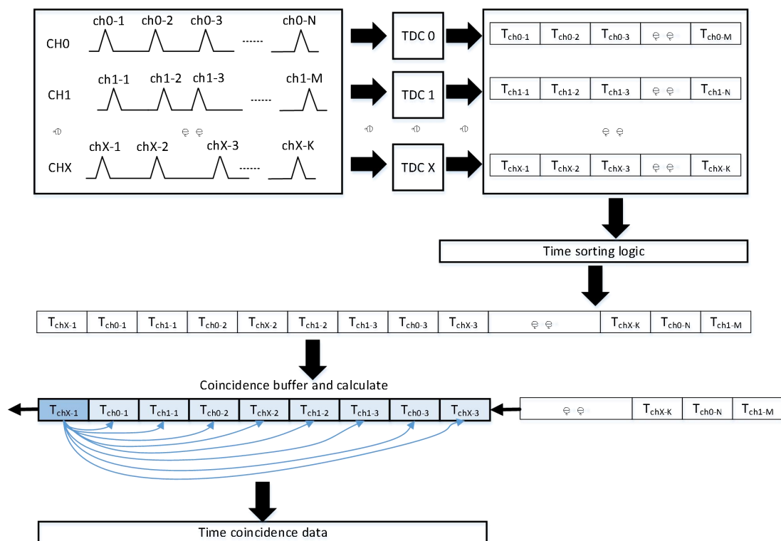
图 147 Venus 在线时间符合事件判断逻辑说明
