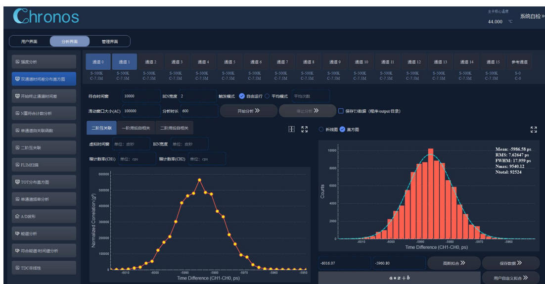
图 110 双通道时间差外部输入信号测量结果（高分辨率通道，通道 0 和 1，上升沿，典型结果）
