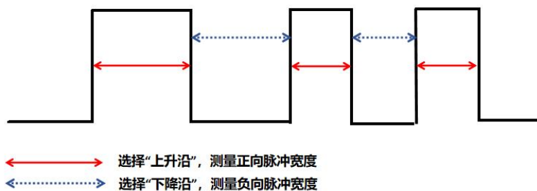
图 40 测量边沿时间戳信息选择举例（选择“上升沿”，TOT 测量中测量正向脉冲宽度；选择“下降沿”，TOT 测量中测量负向脉冲宽度。）
