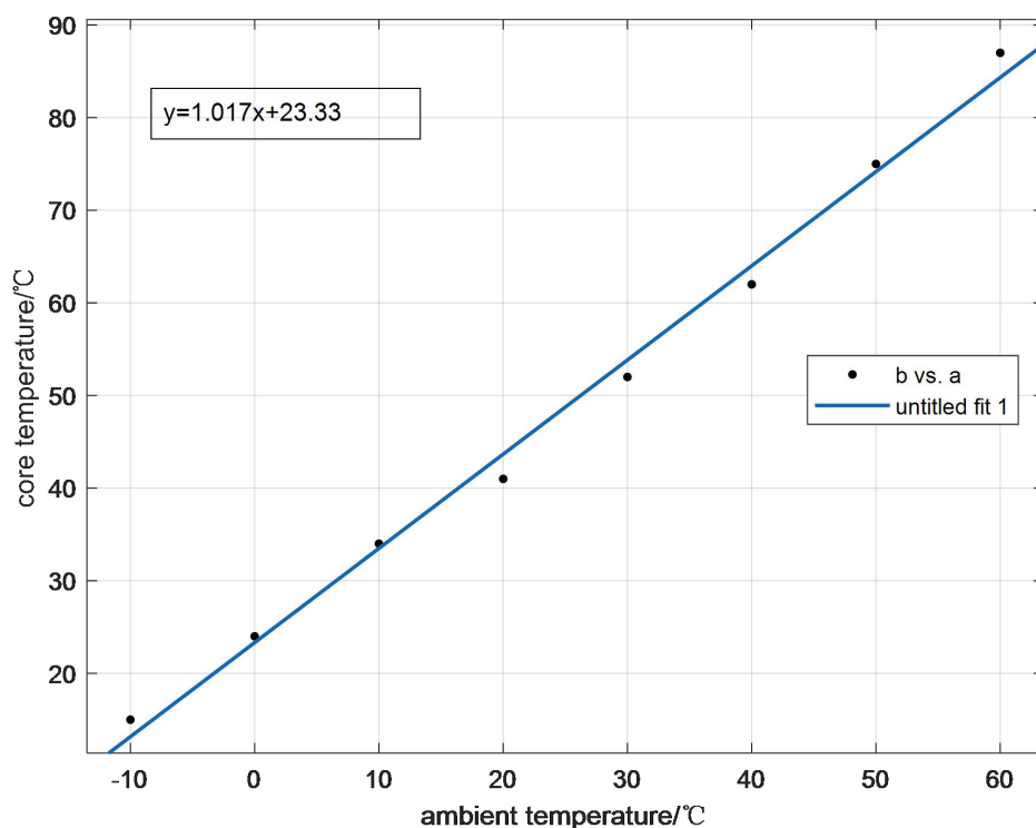
图 132 环境温度与 FPGA 内核稳定温度典型测试结果（Venus lite-T）
