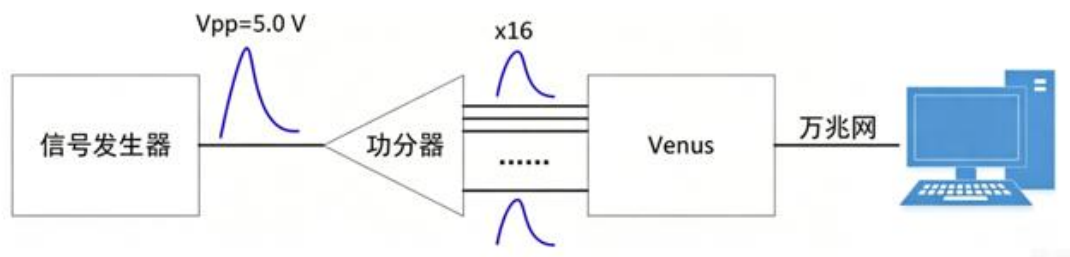
图 109 双通道时间差测量示意图
