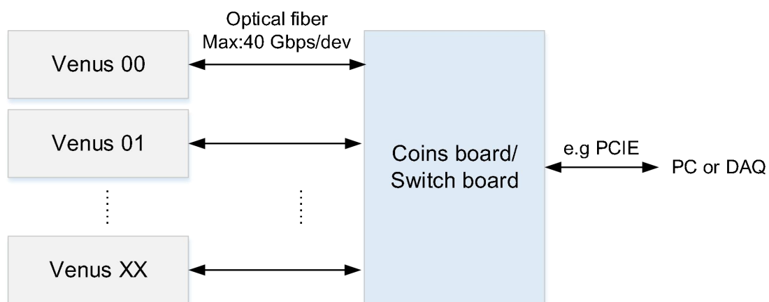
图 144 一种可能的并行数据获取系统架构
