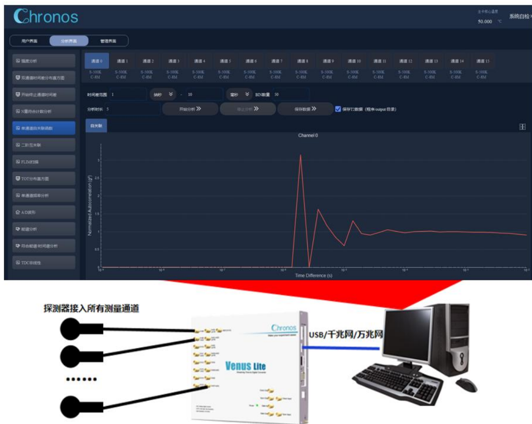
图 69 二阶自关联函数分析
